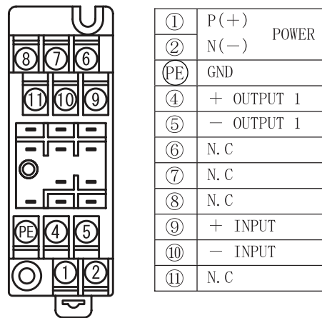
端子配制图、信号布局
